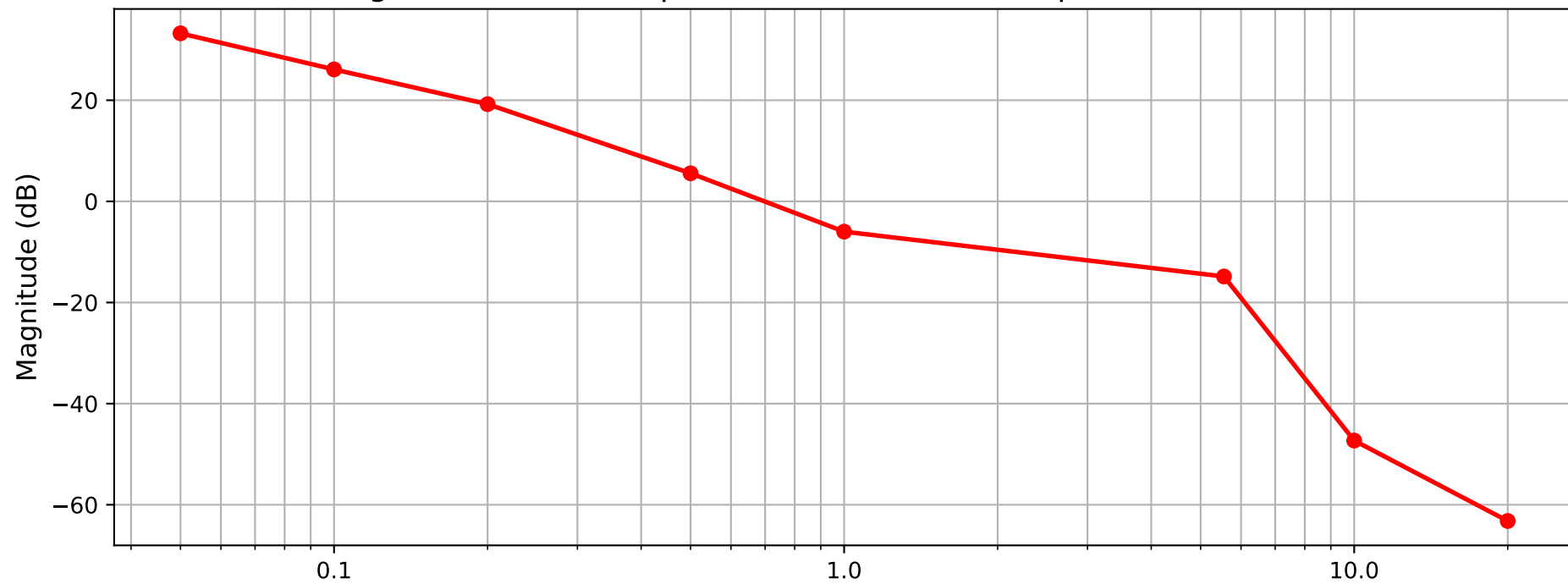
Diagrama de Bode Experimental (Cruzamento por Zero) - Eixo Yaw
